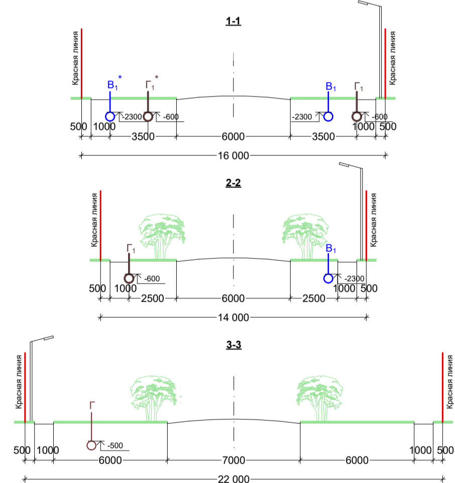
Поперечные профили улиц и дорог Масштаб 1:200
