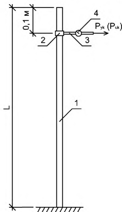
1 — опора; 2 — хомут; 3 — стальной канат; 4 — динамометр; L — длина опоры; P_{yk} — контрольная испытательная нагрузка при испытании на жесткость; P_{ук} — контрольная испытательная нагрузка при испытании на прочность
